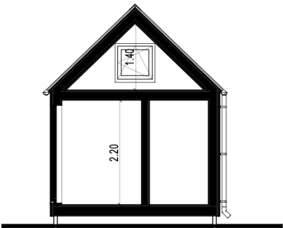
A GRIEZUMS 1:75
