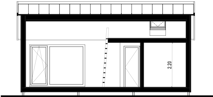
C GRIEZUMS 1:75
