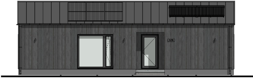
F1 ELEVATION 1:100
